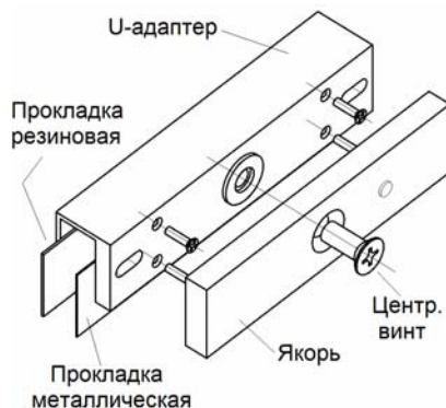
Рисунок 3 – Применение U-адаптера.
